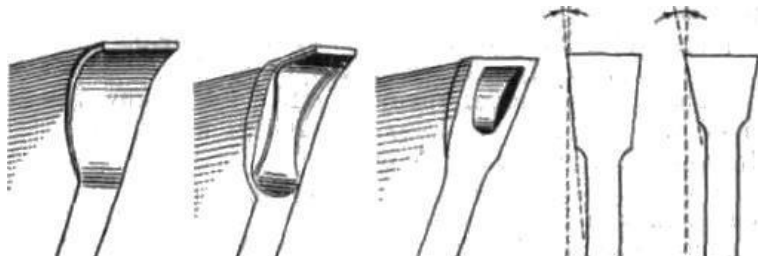
Рекомендовані параметри уширення зуба рамних пил під плющення
