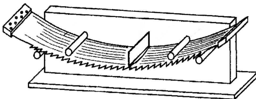
Вальцьована пила повинна мати форму «лодочки»
